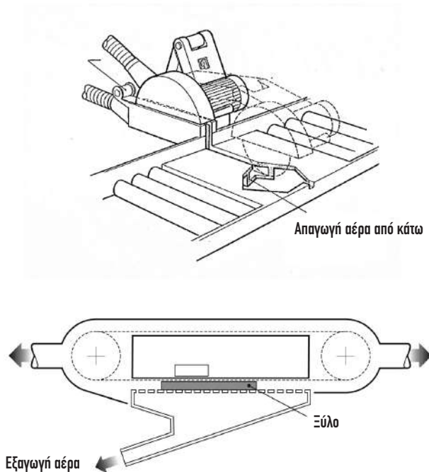
Εικόνα 5. Δίκτυο αεραγωγών και κυλιόμενα απορροφητικά για την απαγωγή της σκόνης ξύλου.
